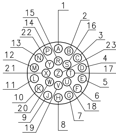
23 pole
